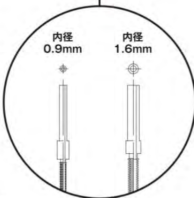
原寸図
